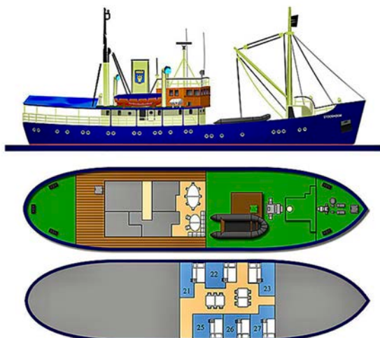
Decksplan mit den 6 Kajüten der „Stockholm“ (blau)
